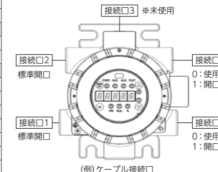
(例)ケーブル接続口
