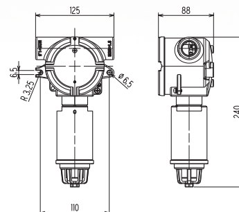
Section du capteur à distance (série GD-3) Modèle par diffusion, avec barrière EC
