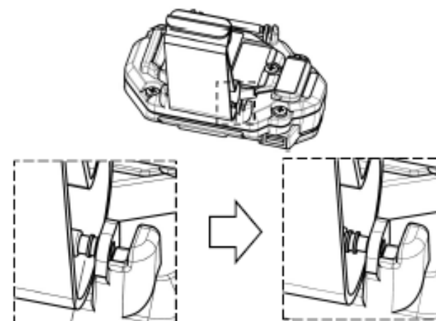
ばね棒の引っ掛け部にマイナスドライバー等を引っ掛け、内側に動かす
