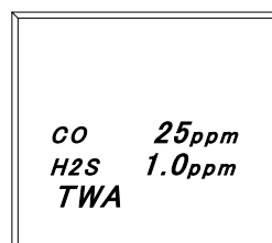
TWA 警报设定值显示
