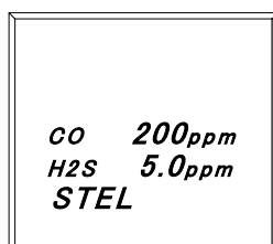
STEL 警报设定值显示
