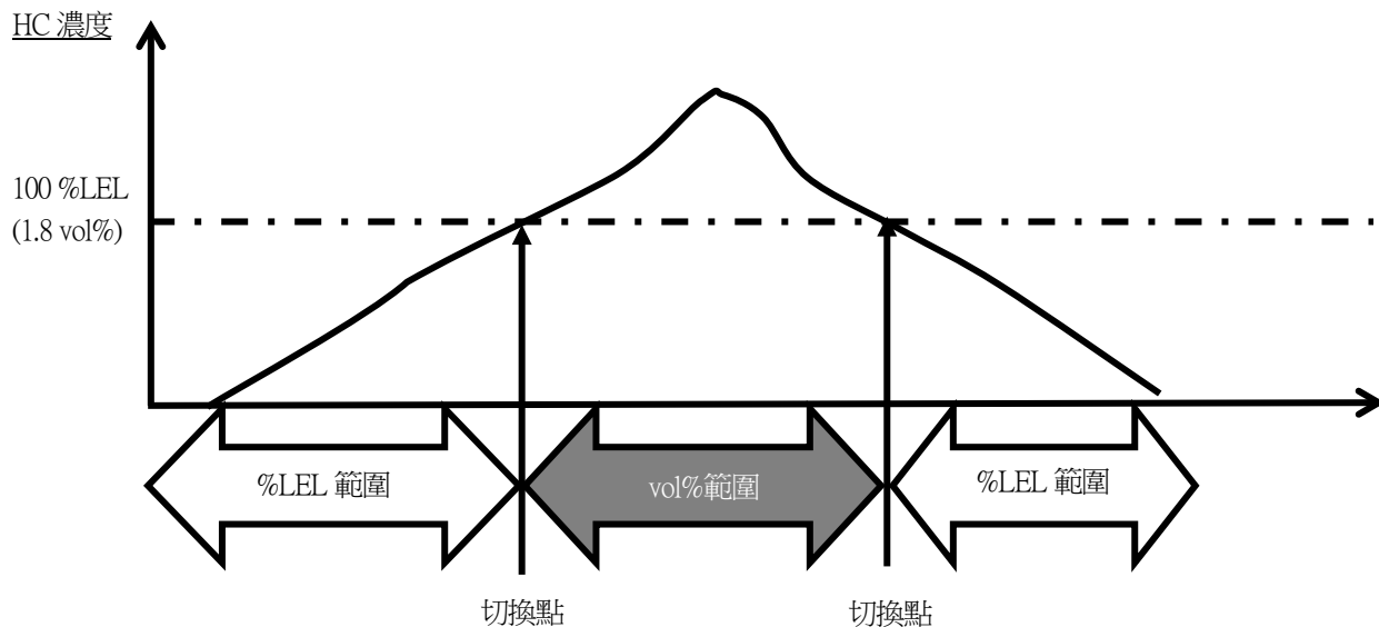
自動範圍的氣體濃度和範圍切換時機圖
