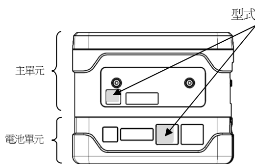
Japan Ex 規格的銘板例
