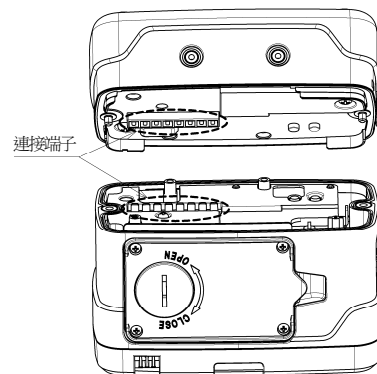
電池單元裝卸螺絲
