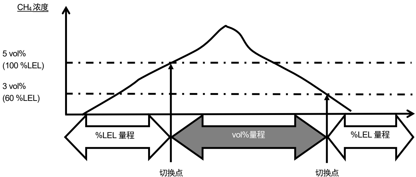
设置为自动量程时气体浓度和量程范围切换时间图
