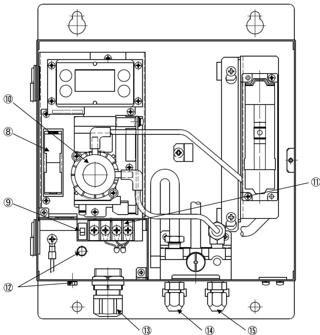
【検知器ユニット前面】
