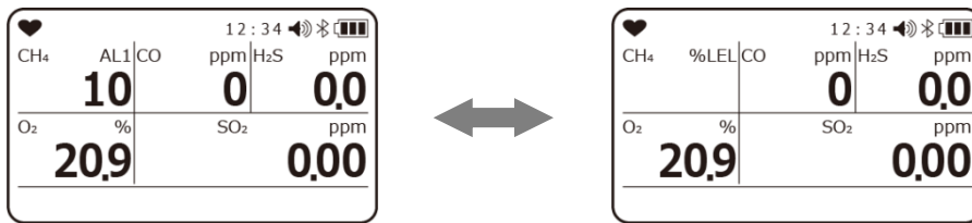
디스플레이 예 메탄 (CH 4 ) 농도: 10%LEL 1 차 알람 작동
