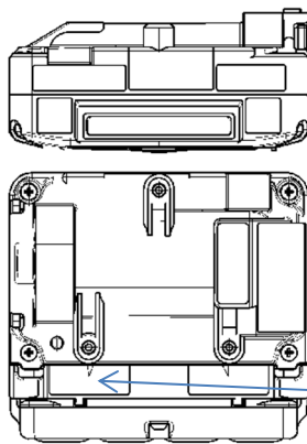
ATEX/IECEx/KCs, CE mark 형식 명판
