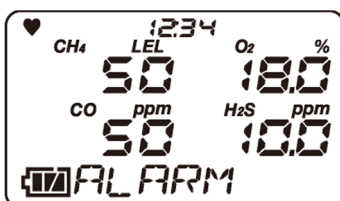
Visor do ponto de ajuste do segundo alarme
