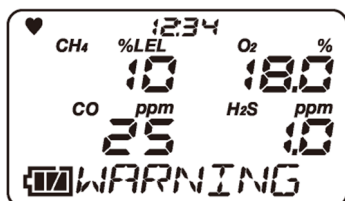
1 차 알람 설정치 화면
