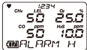
3 차 알람 설정치 화면
