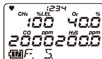
Vollskalen-Anzeige
