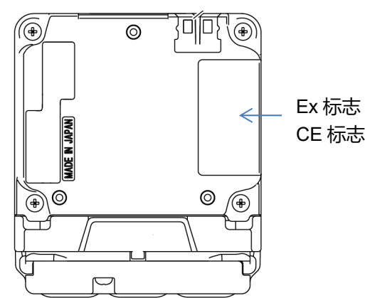
ATEX / IECEx 规格的标牌示例
