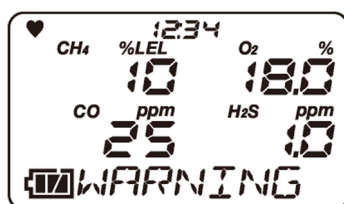
第一警报点显示
