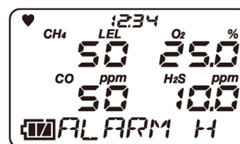
第三警报点显示
