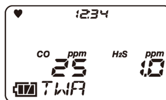
TWA 警报点显示
