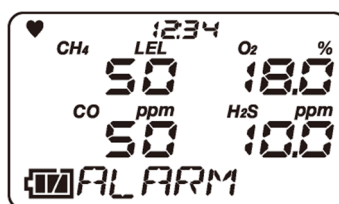
第二警报点显示
