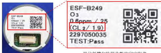
替代氣體和換算係數的印字影像
