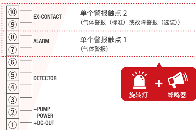
指示器单元接线板布局图
