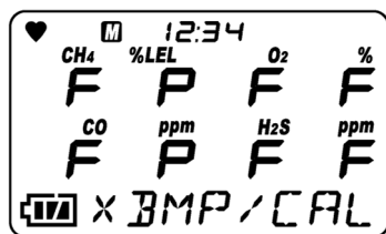
Resultados do teste resposta (ajuste de gás) [P]: Passou, [F]: Falhou
