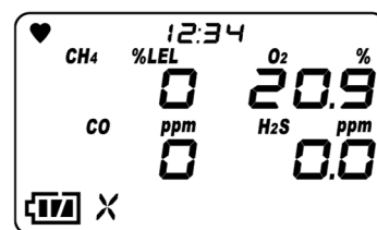
Leituras após o ajuste de gás (Exibido apenas se o ajuste de gás foi realizado)
