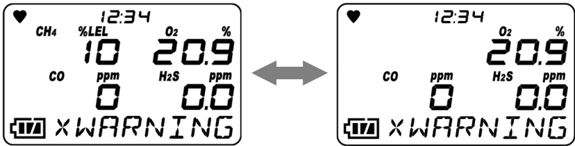
Exemplo de exibição: Concentração de metano CH4: 10 %LEL primeiro alarme acionado
