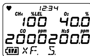
Visor de escala máxima
