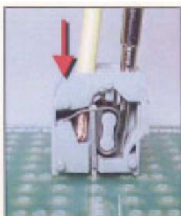
④正しくむき出した電線を電線口(丸穴)に差し込みます。このとき電線を丸穴のフチに沿わせるとスムーズに入ります。
