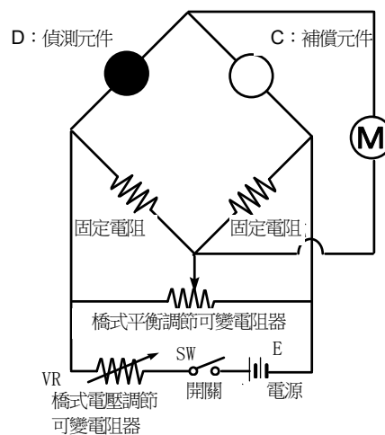
基本電路
