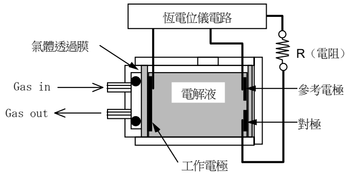
構造圖
