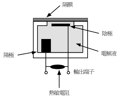
構造圖
