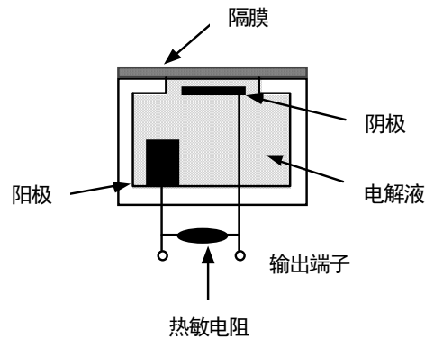
结构图
