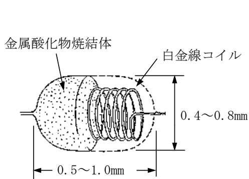
構造図
