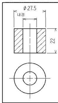
고무 씰
