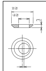
편심 와셔 (재질: SUS303)
