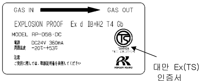
대만 Ex(TS)형 명판 (AC/DC 전원 사양)
