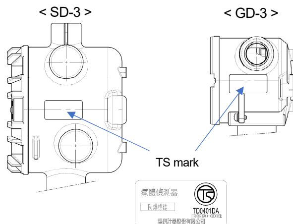
Taiwan Ex(TS)仕様の銘板貼付位置
