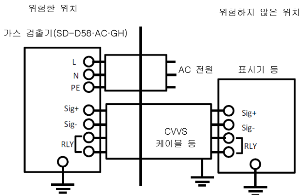
설치 다이어그램
