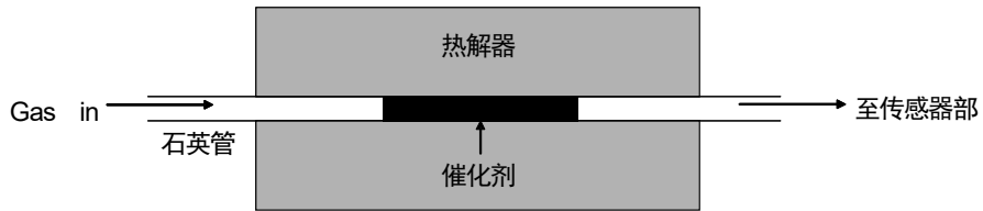
热分解器结构图
