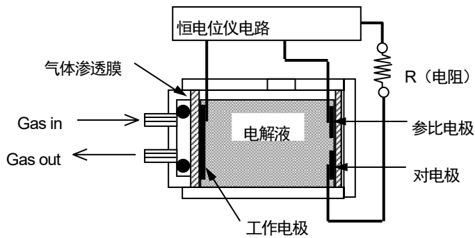
传感器部结构图
