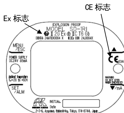
ATEX/IECEX, CE 标志规格的铭牌示例
