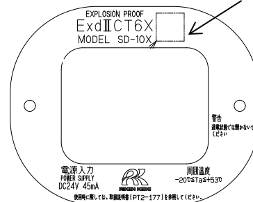
Placa do nome do tipo TIIS
