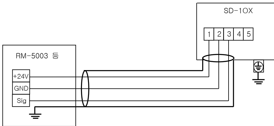
상위 장치에 연결(DCS, PLC)
