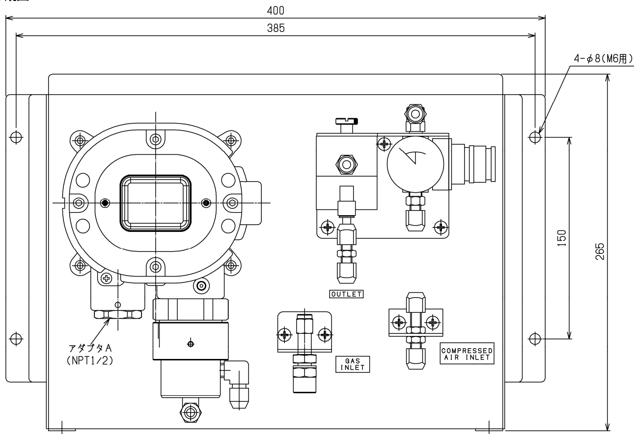
外観図
