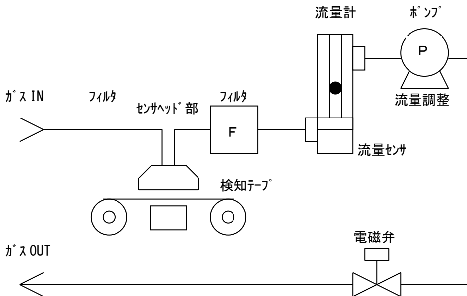
配管図
