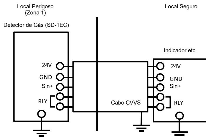
Diagrama de instalação
