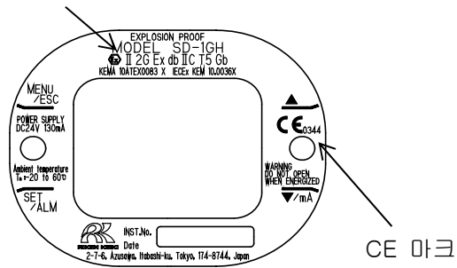
방폭 마킹
