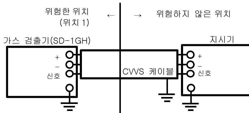
설치 다이어그램
