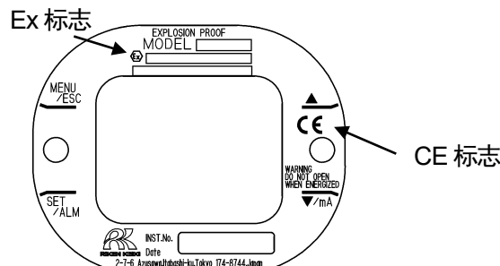
ATEX/IECEX, CE 标志规格的铭牌例
