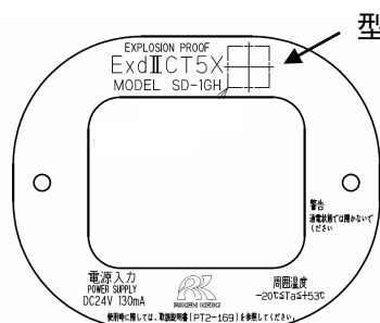
TIIS 规格的铭牌例
