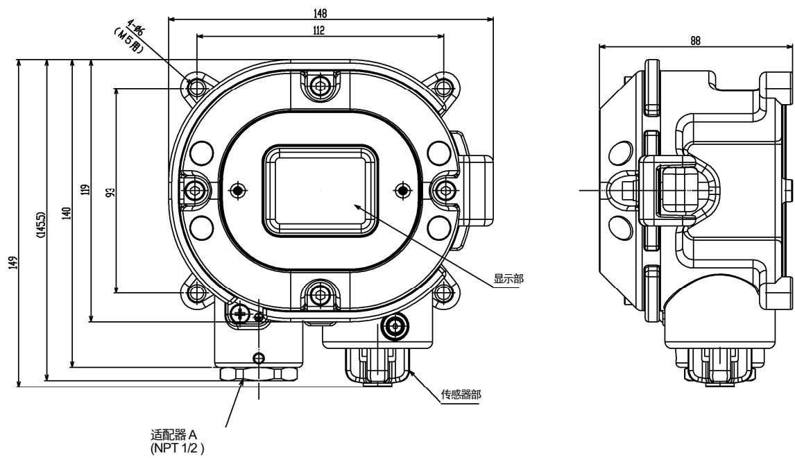
外观图
