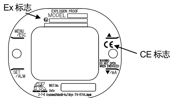
ATEX/IECEx, CE 标志规格的铭牌例
