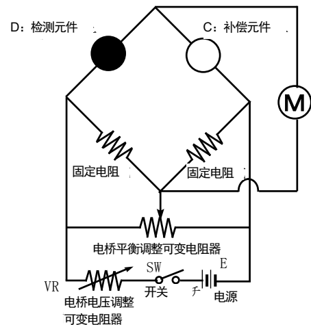
基本回路
