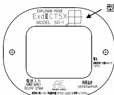
TIIS 规格的铭牌例
