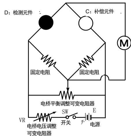
基本回路
