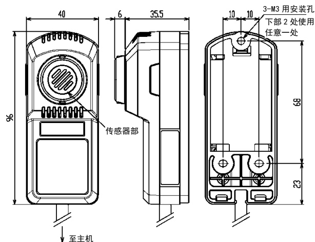
遥控传感器部
