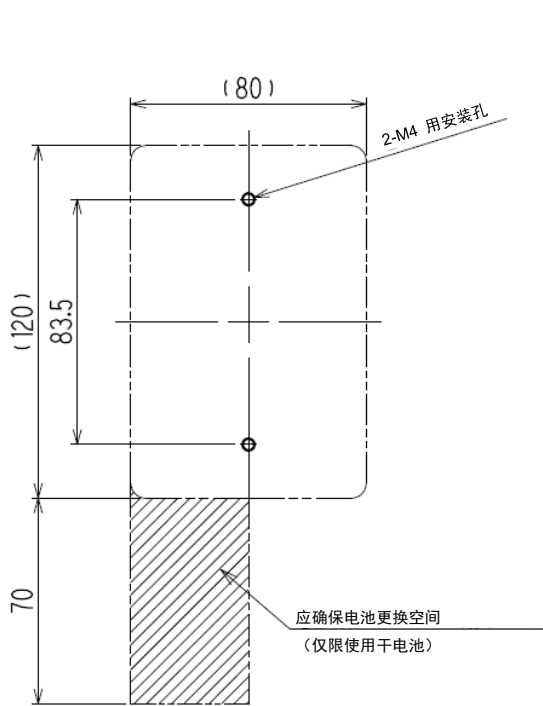
安装尺寸图（未使用安装板） 适合 JIS 1 个用开关盒
