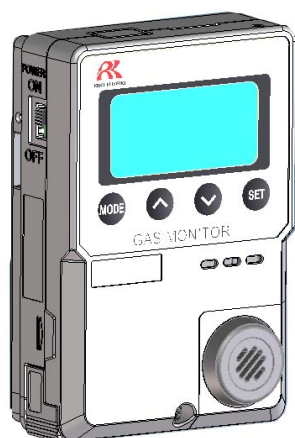
EC-600 本体
