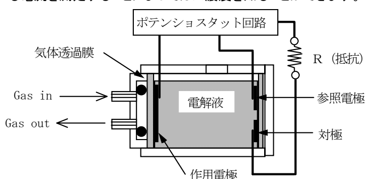
構造図
