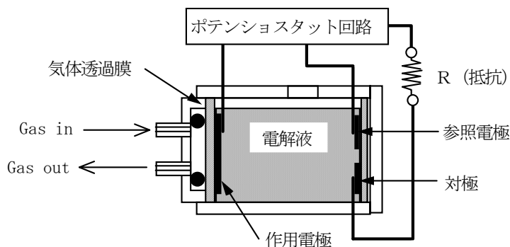
構造図
