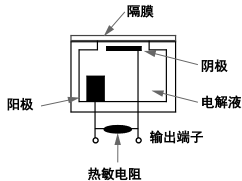
<结构图>
