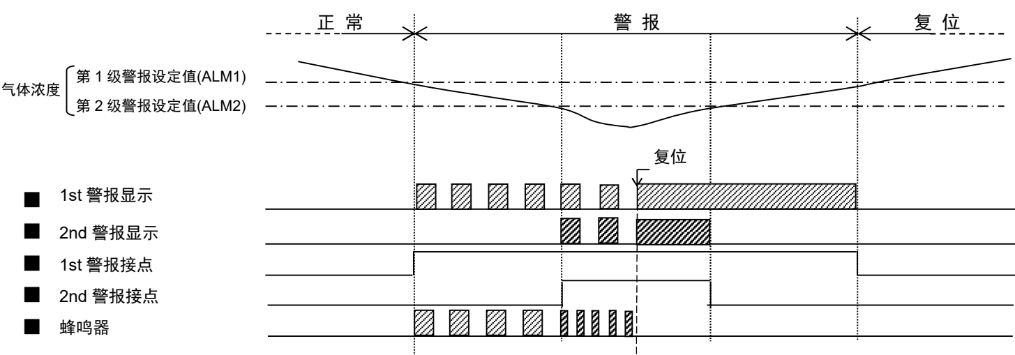
“警报模式示例（自我保持，L-LL）”
