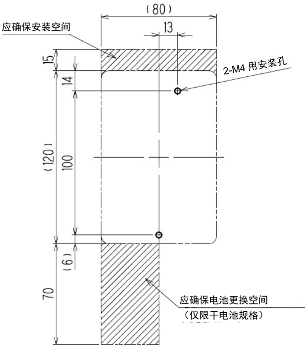
安装尺寸图（使用安装板）
