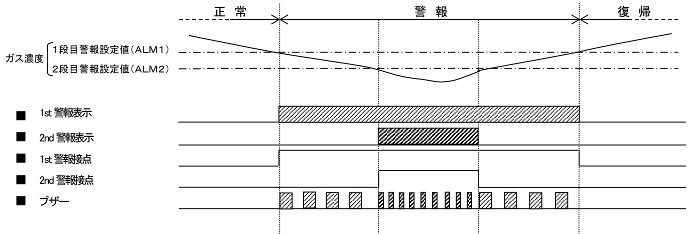
『警報パターン例(自動復帰,L-LL)』
