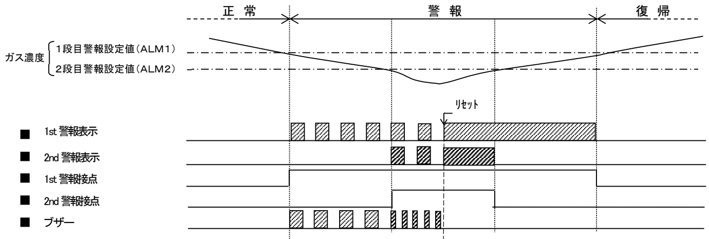
『警報パターン例(自己保持,L-LL)』
