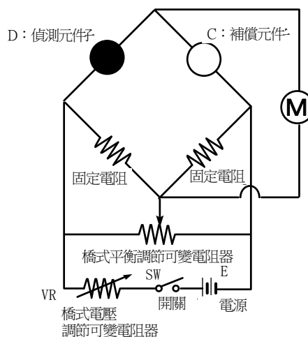
基本電路
