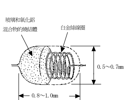
構造圖
