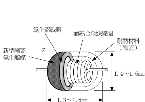
構造圖
