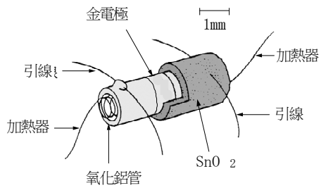
構造圖
