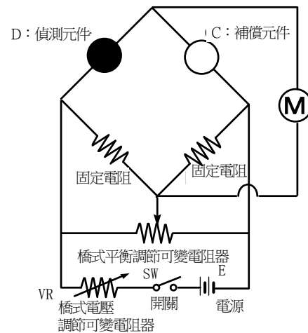
基本電路
