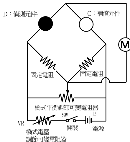
基本電路
