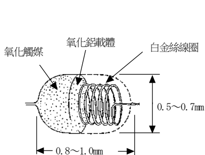
構造圖
