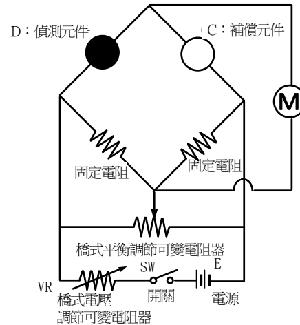
基本電路
