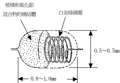
構造圖
