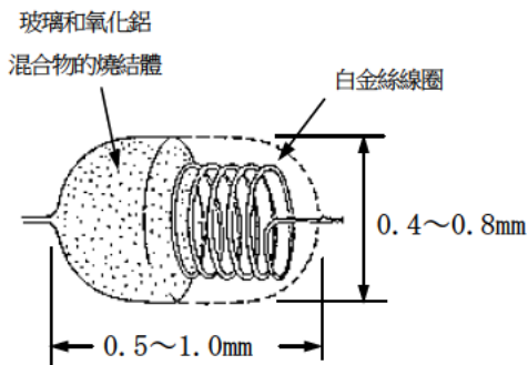
構造圖
