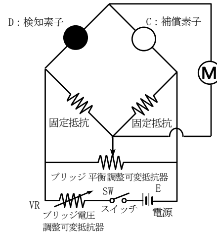
基本回路
