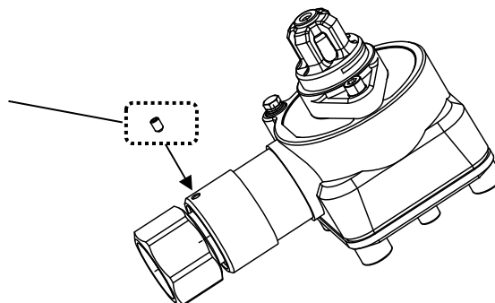
六角穴付き止めネジ M4 × 6
