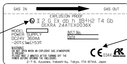
ATEX, CE マーキング仕様の銘板例 (DC 電源仕様のみ)
