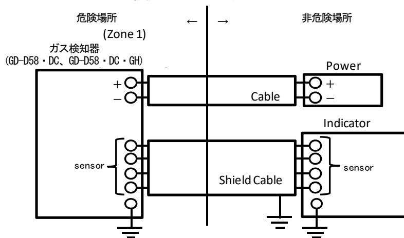
接続図 (GD-D58・DC、GD-D58・DC・GH)
