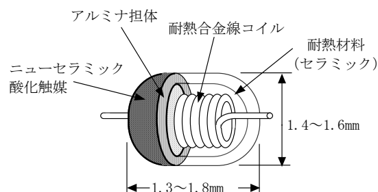
構造図
